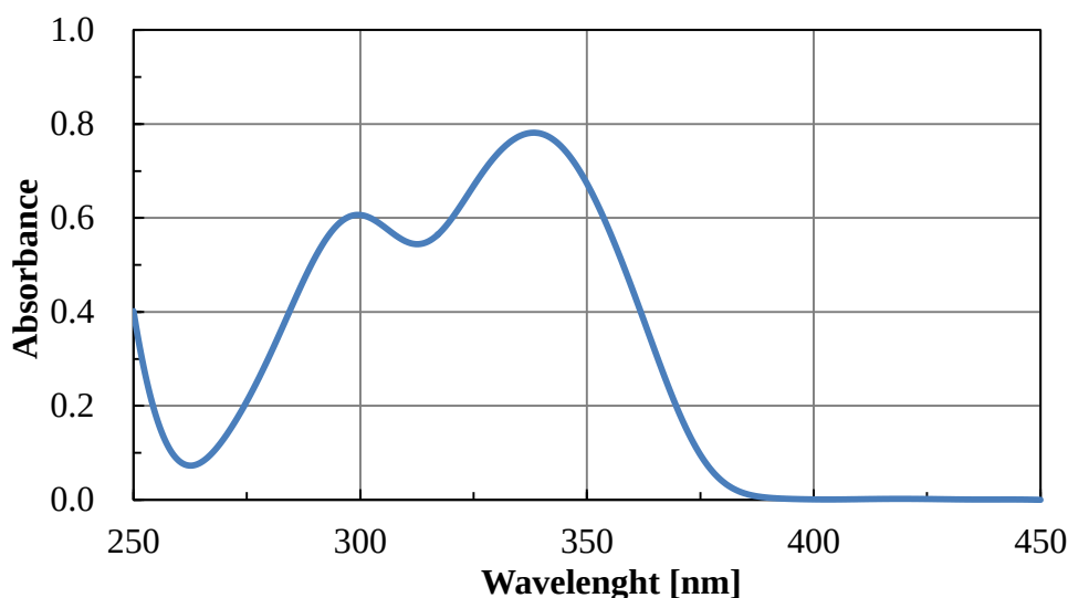
UVA-101~104 紫外線吸収スペクトル
