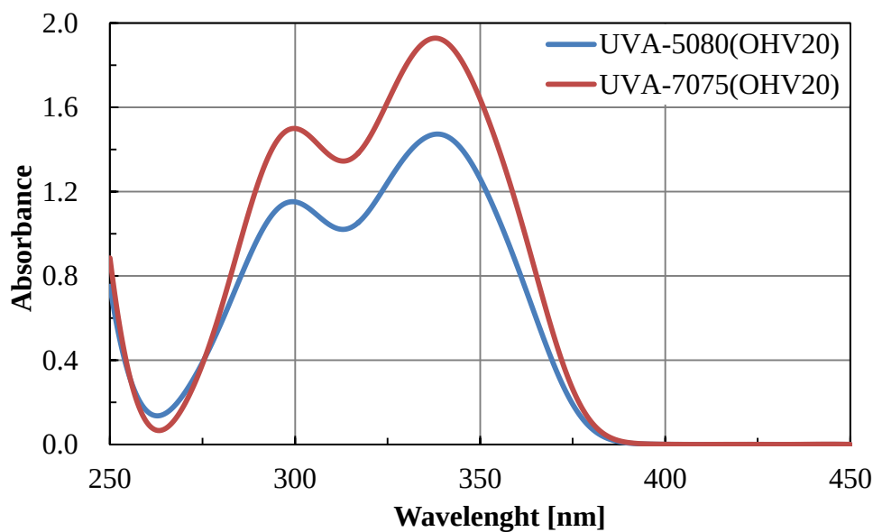
紫外線吸収スペクトル
